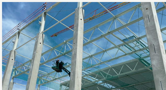
Personen-Auffangnetz horizontal auf Grossbaustelle
