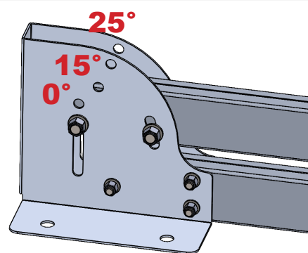
0° / 15° / 25° Neigung
